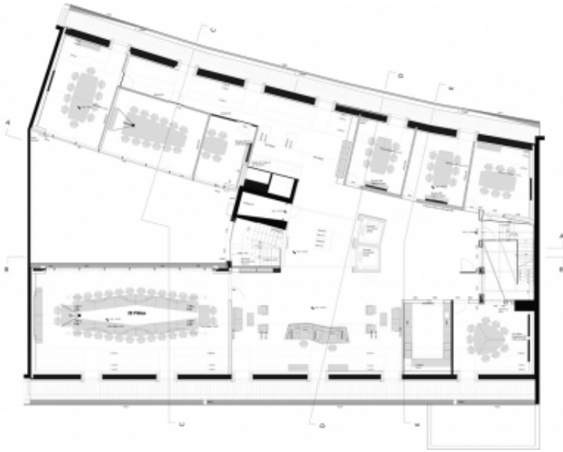
Grundriss Dachgeschoss
